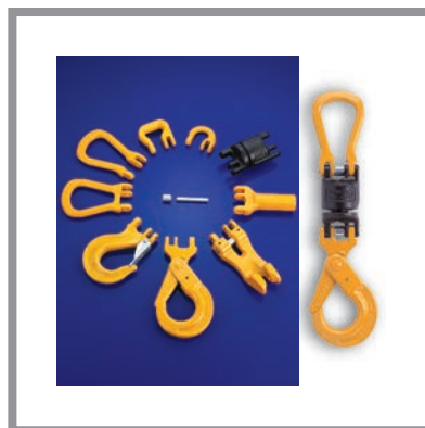
Isolierdrallfänger - kugelgelagert Insulated Swivel - ball bearing
